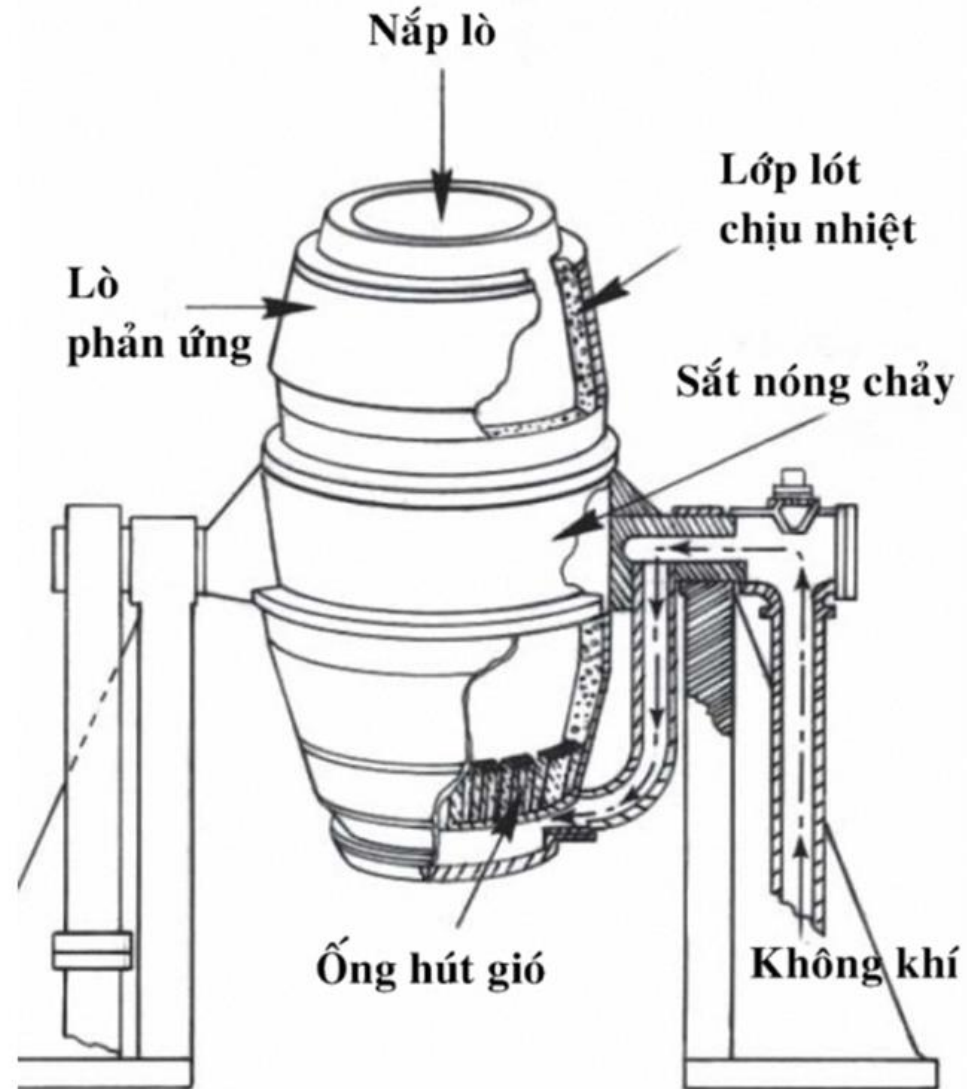
Lò sản xuất thép của Henry Bessemer. Ảnh: Chemical Engineer.
